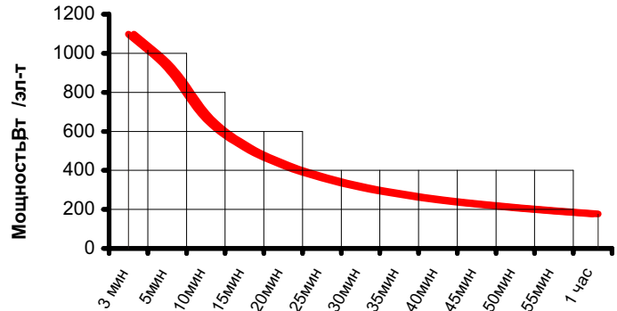
Разряд постоянной мощностью U_{кон} = 1.7 \text{ В/эл-т} T = 20^\circ\text{C}
